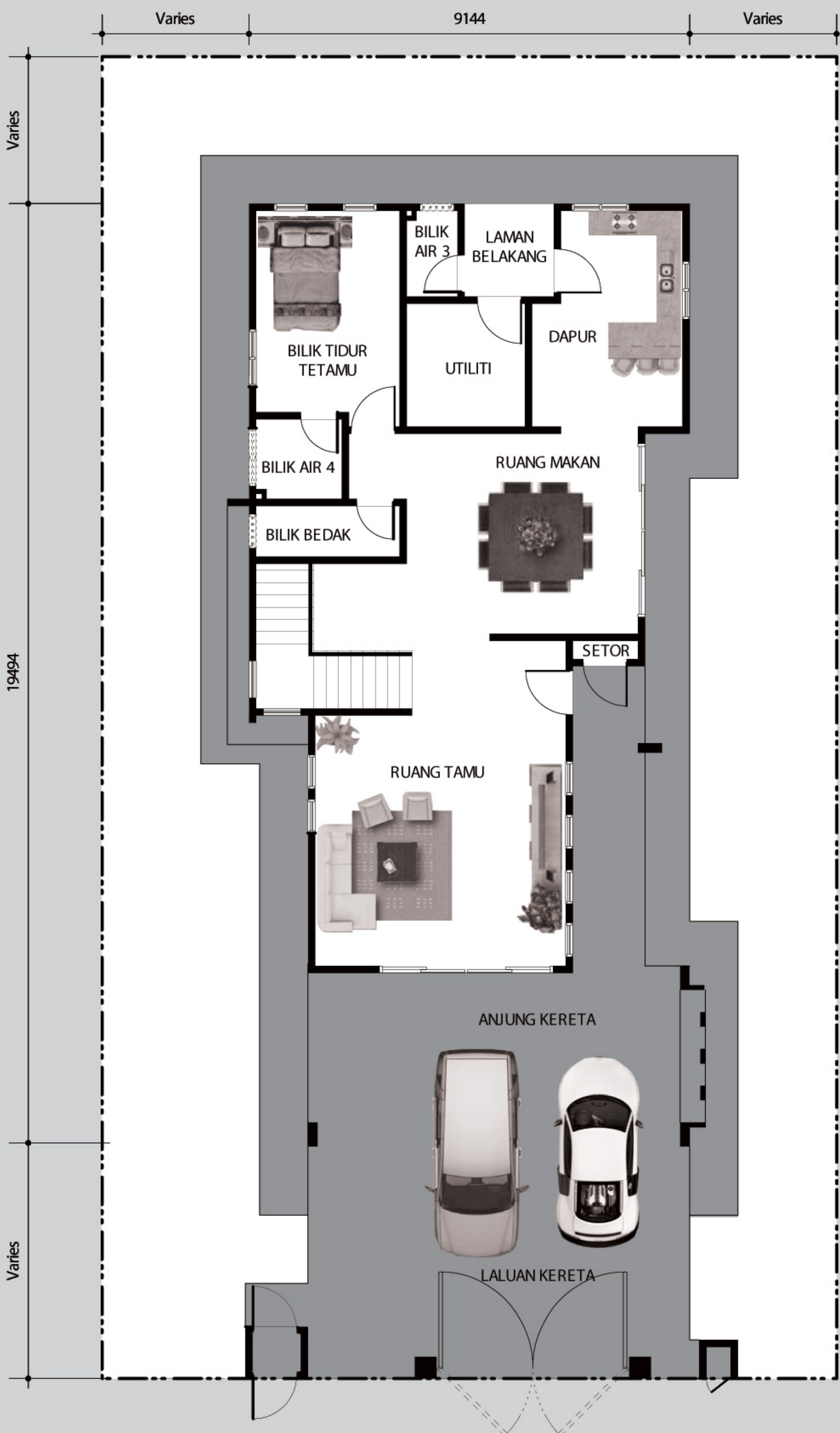
TINGKAT BAWAH
