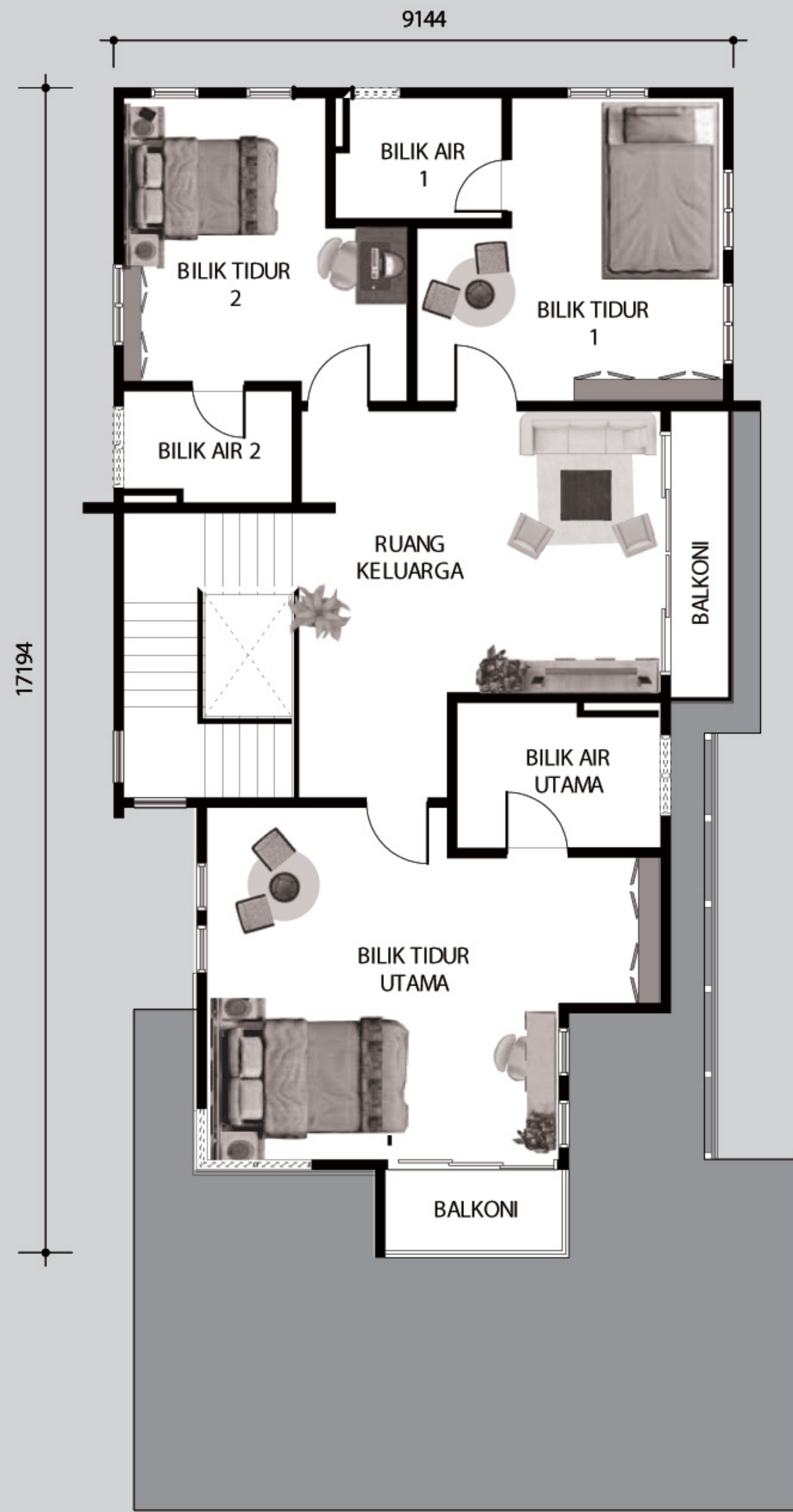
TINGKAT ATAS
